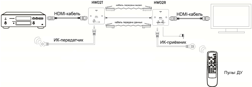
Рис. 3 Схема подключения
