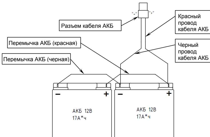
Рисунок 5 – схема параллельного соединения двух АКБ
