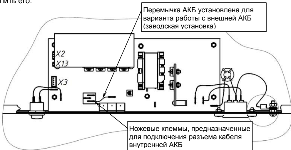
Рисунок 3 – вид на плату источника
