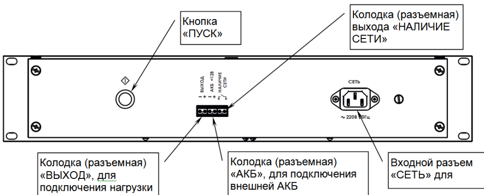
Рисунок 2 – задняя панель источника
