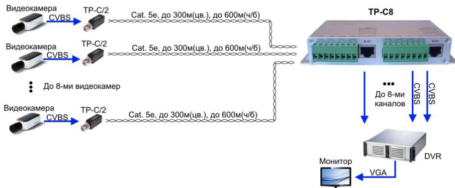
Рис.2 Схема подключения TP-C8
