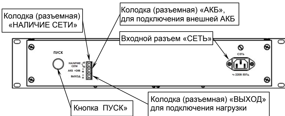
Рисунок 2 – задняя панель источника
