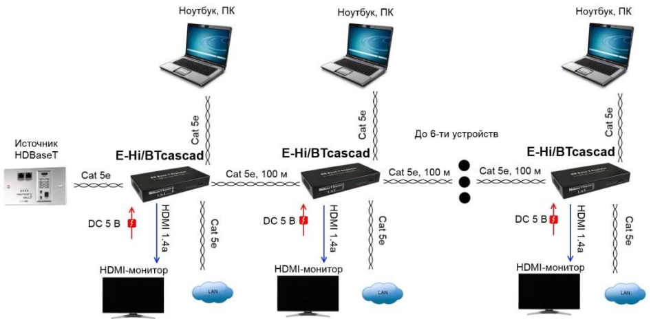
Рис. 4 Схема подключения E-Hi/VTcascad
