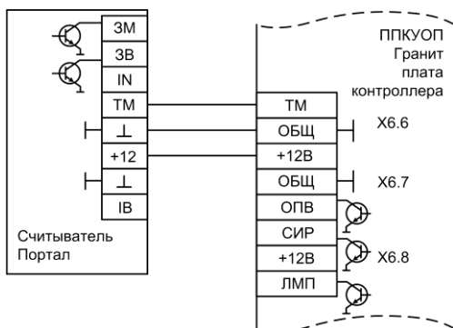
Рис.Б4 Схема подключения считывателя «Портал»
