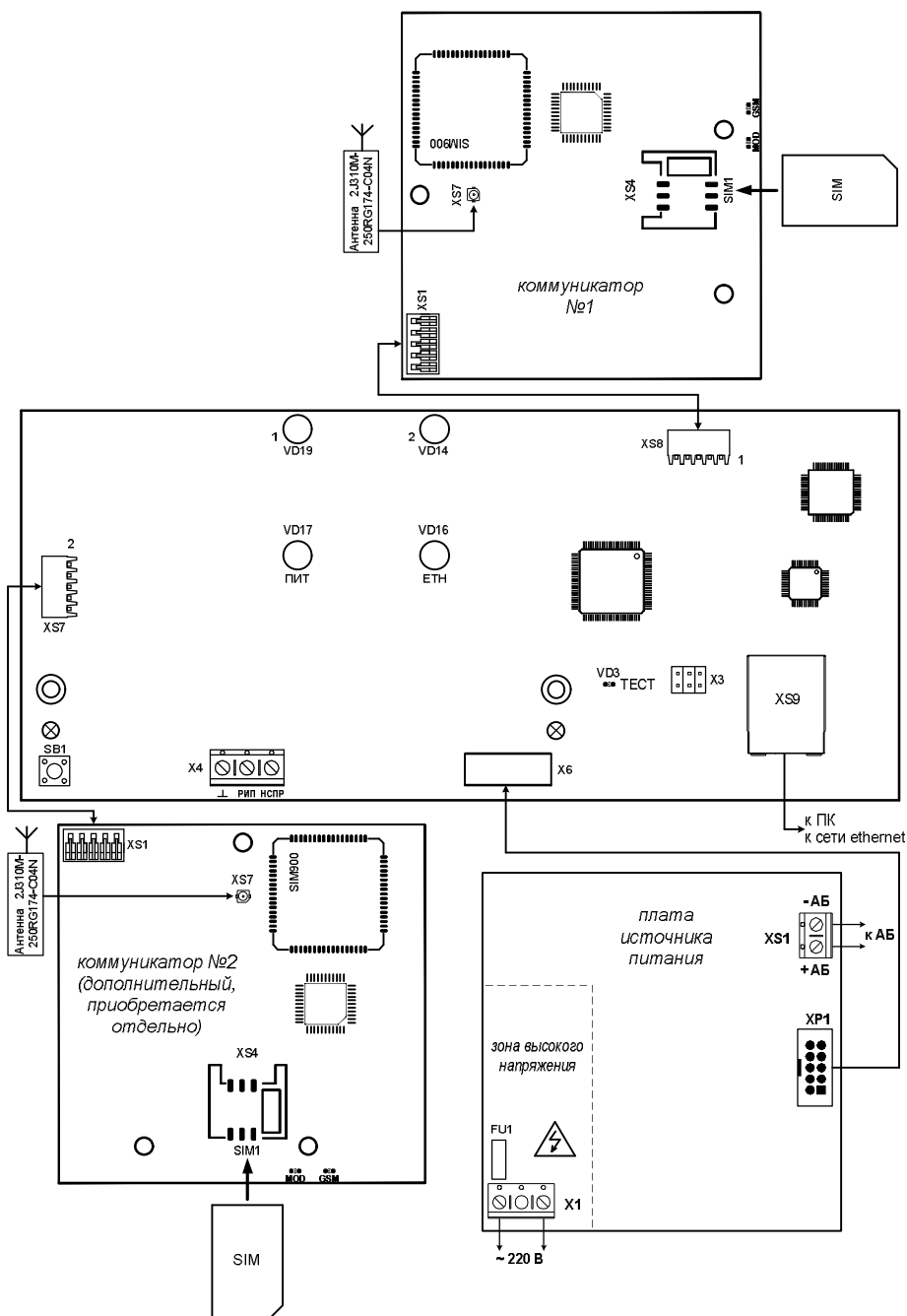
Рис.9 Схема соединений
