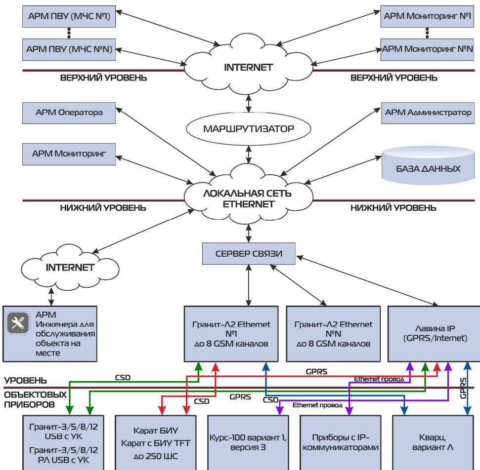
Рис.1 Структурная схема системы «ЛАВИНА»
