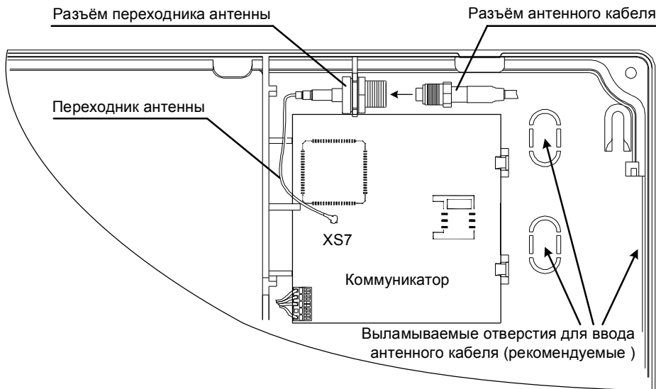
Рис. 8 Подключение антенны к переходнику
