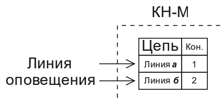
Рис.1. Схема подключения линии к согласующей коробке «КН-М».
