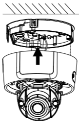
Рисунок 2-10 Закрепите корпус камеры
