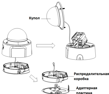
Рисунок 2-2 Разбор камеры
