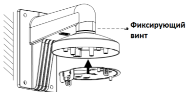
Рисунок 2-14 Установка адаптерной пластины на кронштейн
