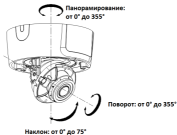
Рисунок 2-12 Настройка углов наблюдения
