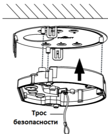
Рисунок 2-8 Установка распределительной коробки
