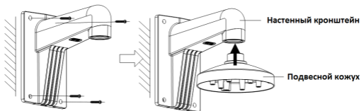
Рисунок 2-13 Установка настенного кронштейна
