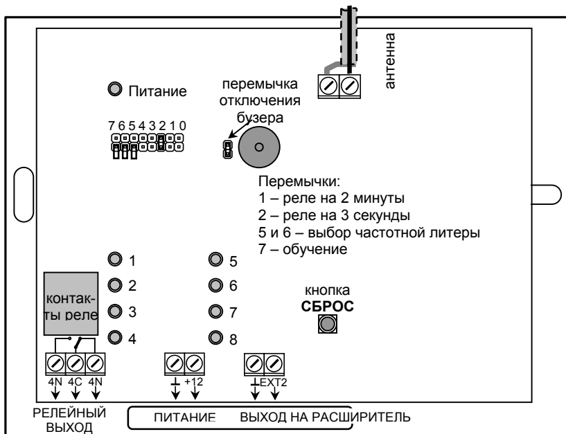
Рис. 3. Монтажная схема приёмника
