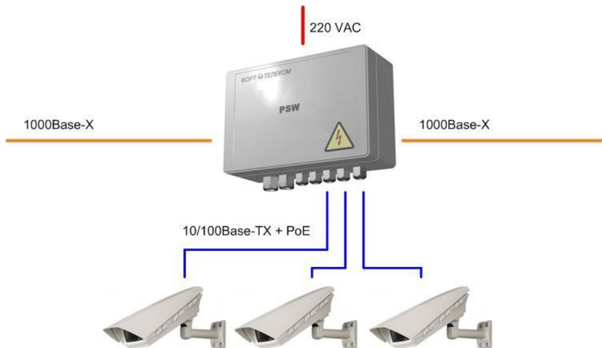
Рис. 1. Схема подключения PSW-2G
