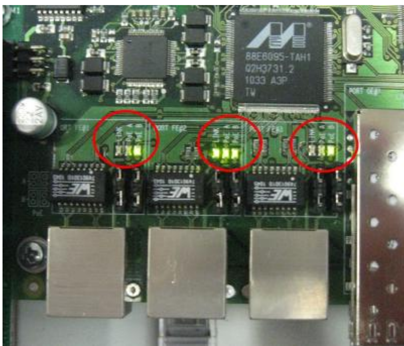
Рис. 2.7.1-3. Индикатор LINK, PoE «A», PoE «B» на порту FE
