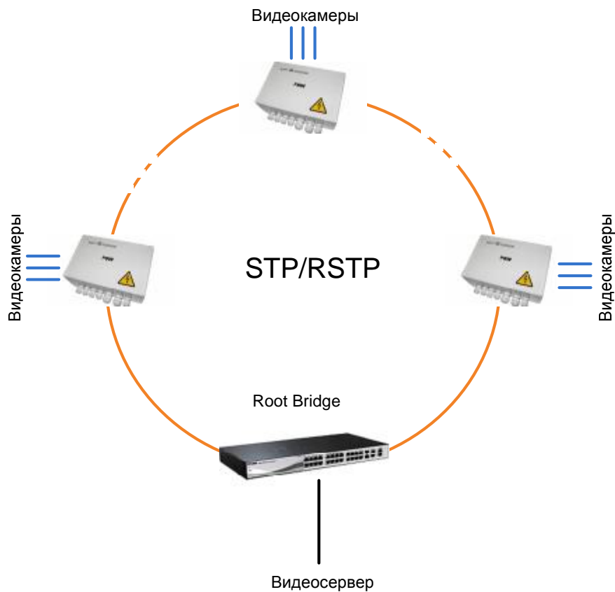
Рис. 2.3-5. Топология «Кольцо»
