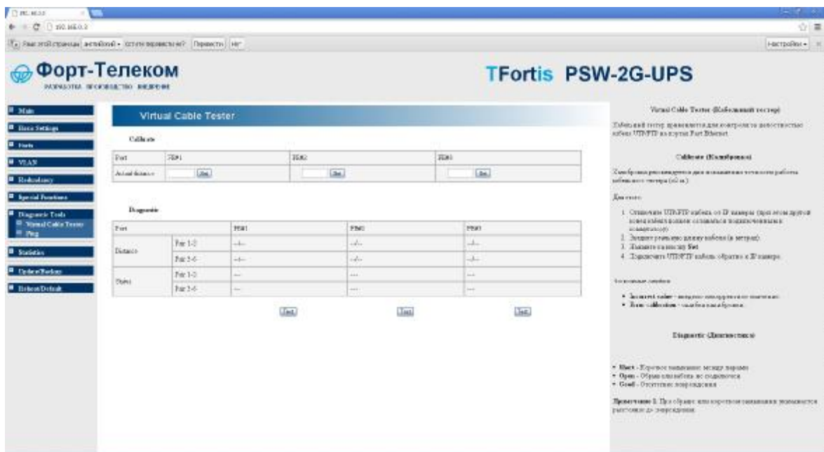
Рис. 7.7.1. Virtual Cable Tester (Виртуальный кабельный тестер)
