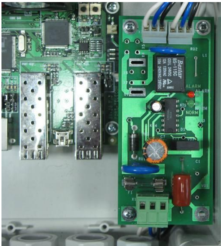
Рис. 2.10. Реле контроля напряжения
