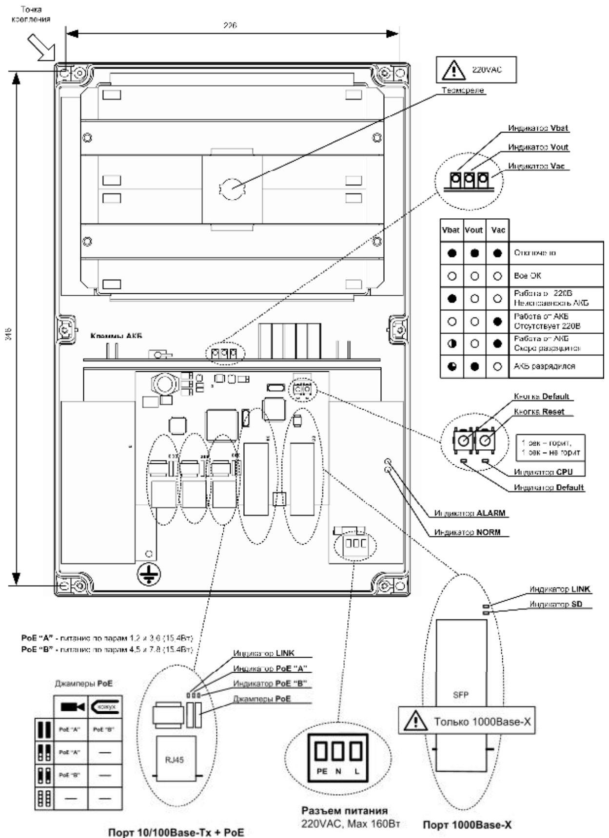
Рис. 2.7-2. Расположение элементов PSW -2G-UPS
