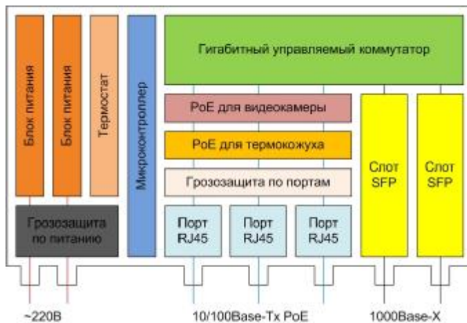
Рис. 2.2-1. Структурная схема блока PSW-2G.
