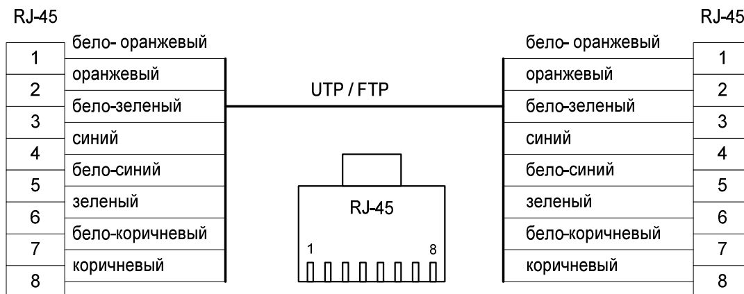
Рис. 6.2. Разделка UTP/FTP кабеля.
