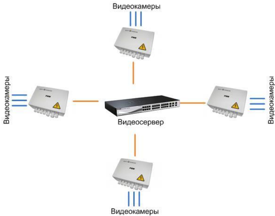
Рис. 2.3-3. Топология «Звезда».
