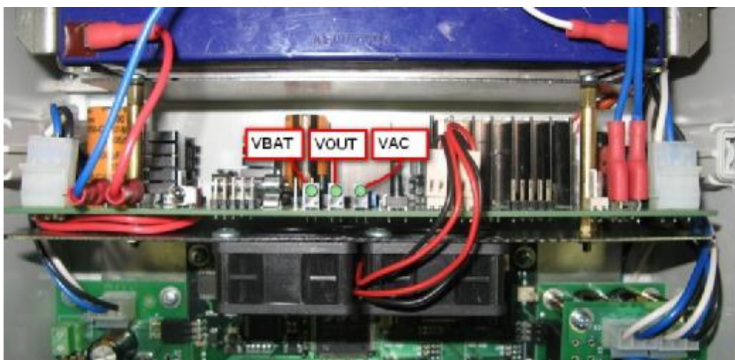
Рис. 2.11. Узел встроенного источника бесперебойного питания
