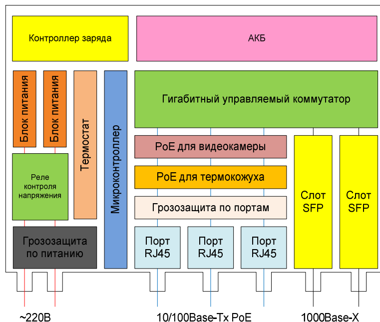
Рис. 2.2-2. Структурная схема блока PSW-2G-UPS.
