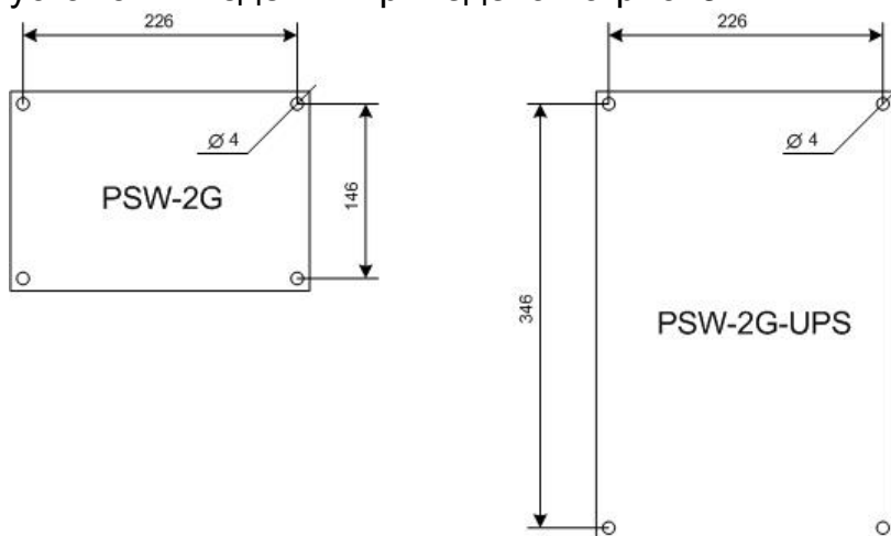
Рис. 5.1. Разметка крепления
