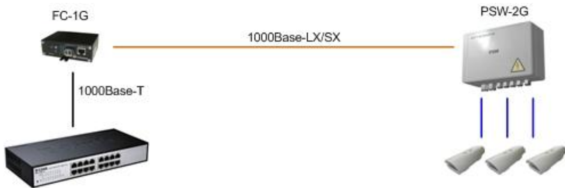
Рис. 2.3-6. Подключение PSW-2G с помощью FC-1G
