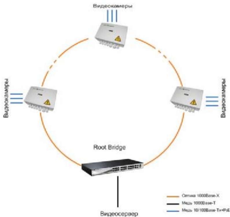
Рис. 7.5. Пример организации системы видеонаблюдения с резервированием.
