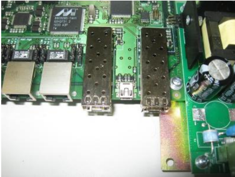
Рис. 2.3-1. Порты GE.
