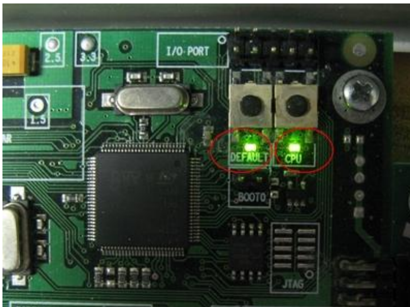
Рис. 2.7.1-5. Индикатор CPU и DEFAULT
