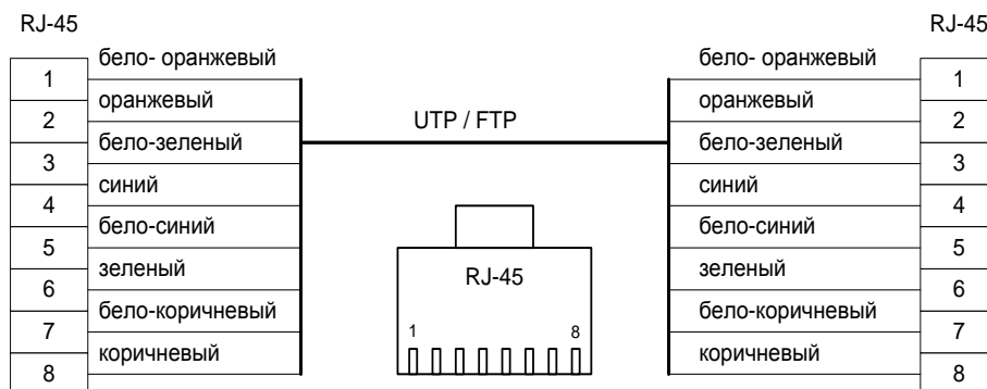
Рис. 6.4. Разделка UTP/FTP кабеля.
