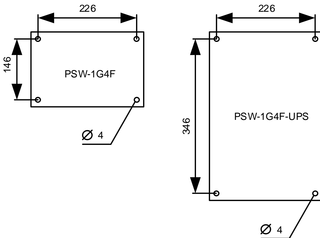
Рис. 6.1.1. Разметка крепления
