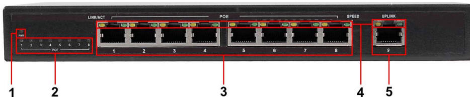
Рис. 2 Коммутатор SW-20900/B, разъемы и индикаторы на передней панели
