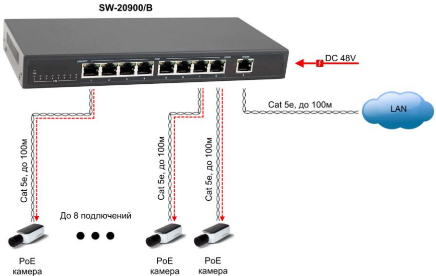
Рис.4 Типовая схема подключения коммутатора SW-20900/B
