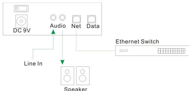
Рис.3.1. Схема подключения LPA-8502NAS
